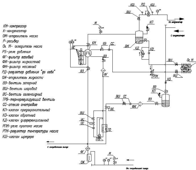
Стандартная комплектация агрегата
