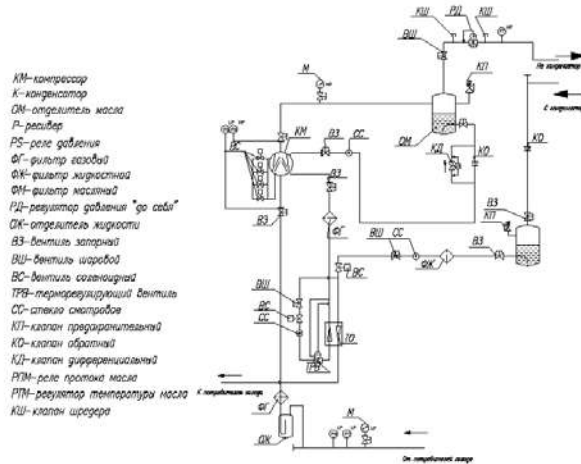
Стандартная комплектация агрегата
